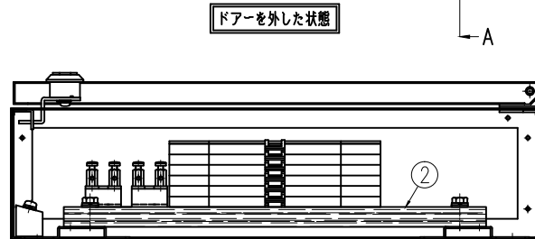
断面 BB
