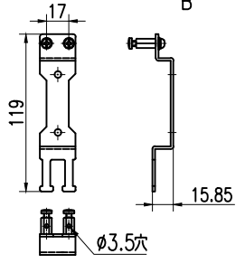
ケーブルホルダ詳細図
