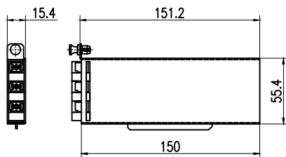
WDMモジュール外観図
