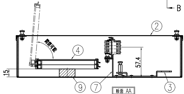
コードホルダ詳細図 (添付品)
