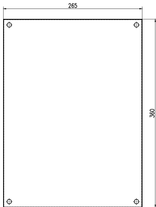
ケーブルホルダ詳細図 ケーブル2条保持可能
