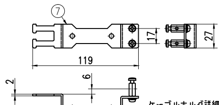
ケーブルホルダ詳細図 ケーブル2条保持可能
