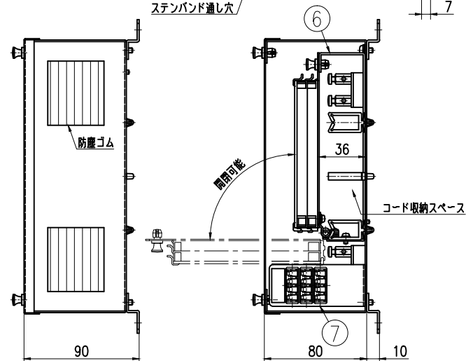
断面 BB
