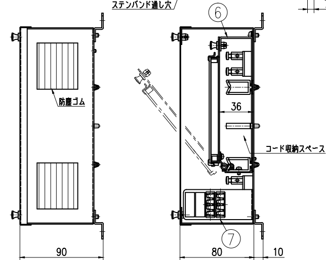
断面 BB
