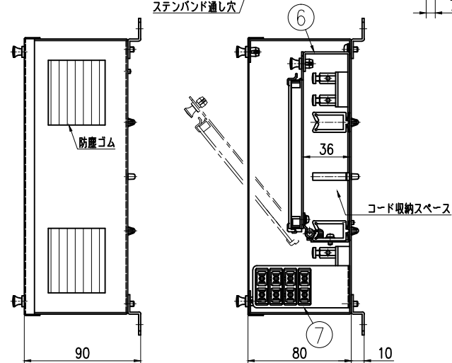
断面 BB
